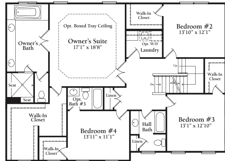
Optional Upper Level Plan
